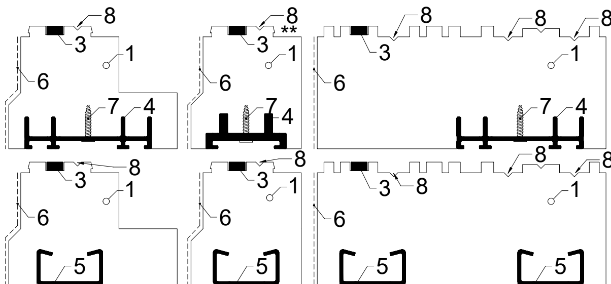
Rysunki poglądowe. Kształt frezowań jest dopasowany do konkretnego systemu.
